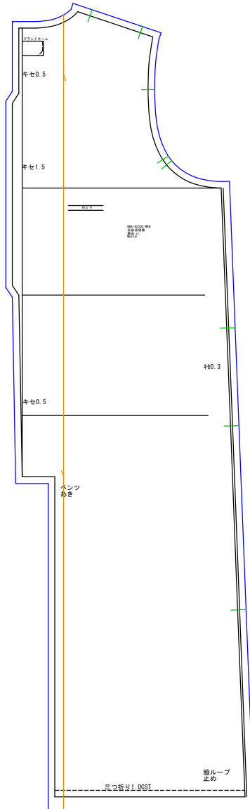
左後身頃裏 (1/8. 1) 裏地x1
