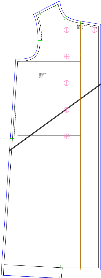
右前身頃 (1/8. 6) 表地x1 芯地x1
