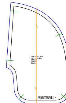
ポケット袋布 表地x2 裏地x2
