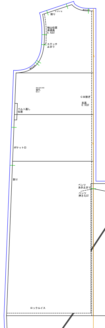
後身頃 (1/8.5) 表地x2
