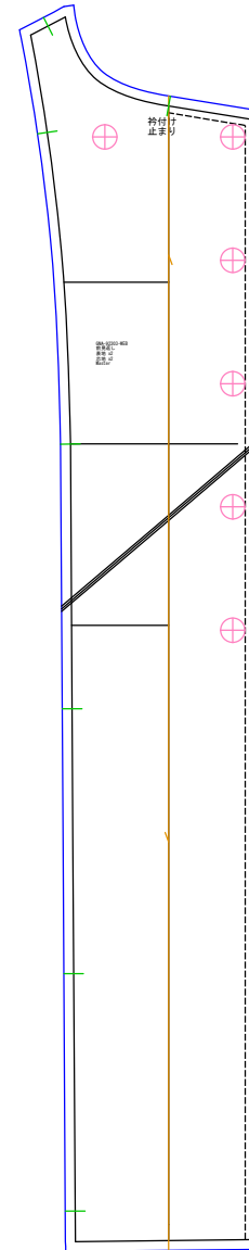
前見返し (1/8. 3) 表地x2 芯地x2
