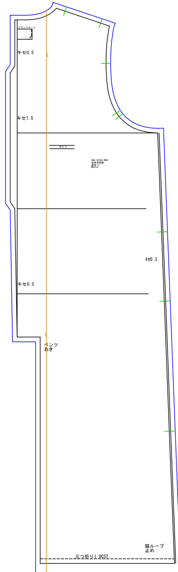
左後身頃裏 (1/8. 1) 裏地x1
