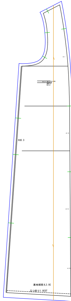
前身頃裏 (1/8. 1) 裏地x2
