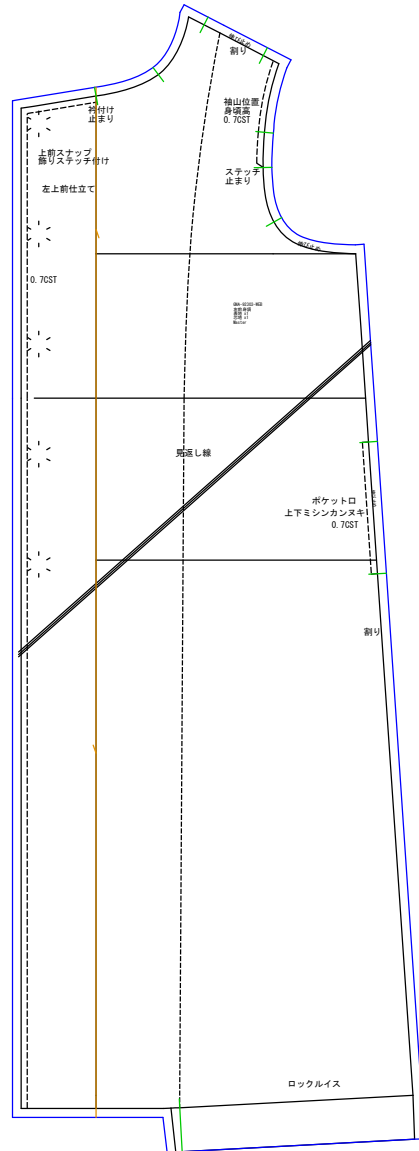
左前身頃 (1/8.6) 表地x1 芯地x1
