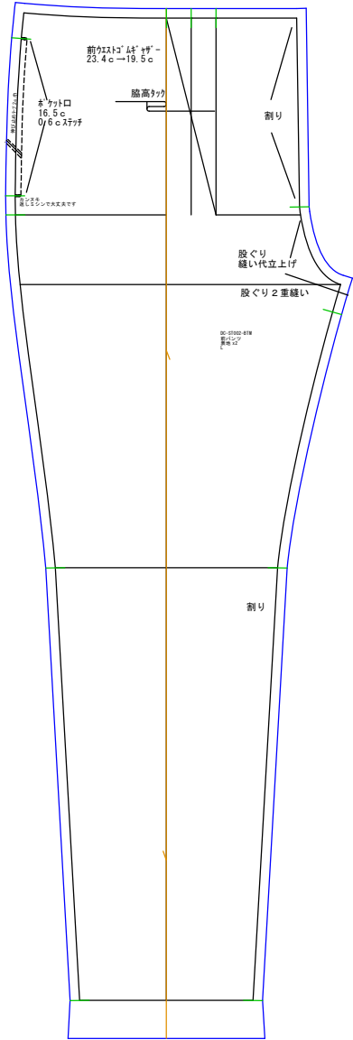
前パンツ (1/7.2) 表地x2
