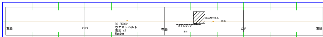
ウエストベルト 表地x1
