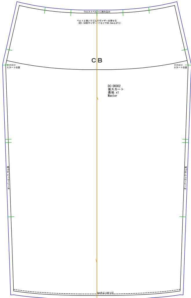
後スカート 表地x1
