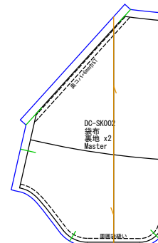
袋布 裏地x2
