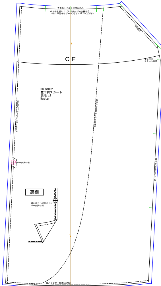
左下前スカート 表地x1
