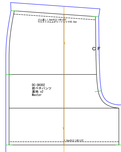
前ペチパンツ 裏地x2
