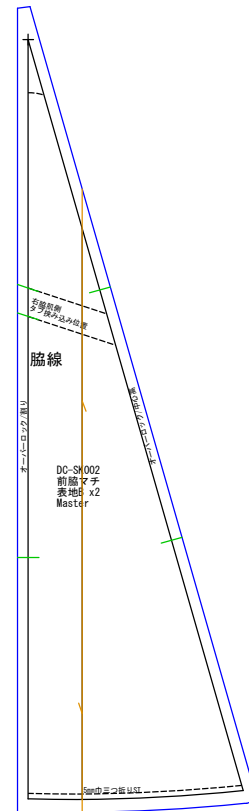
前脇マチ 表地Bx2
