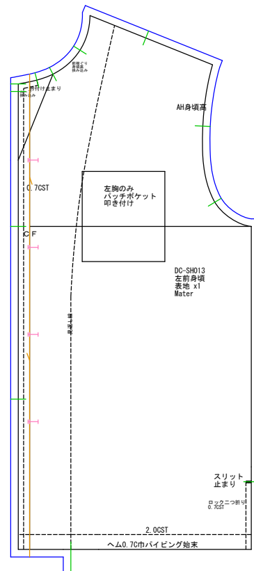
左前身頃 表地x1
