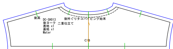
後ヨーク 表地x1 裏地x1
