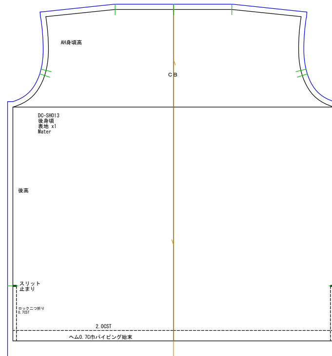
後身頃 表地x1
