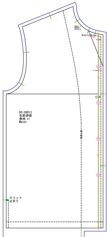
右前身頃 表地x1
