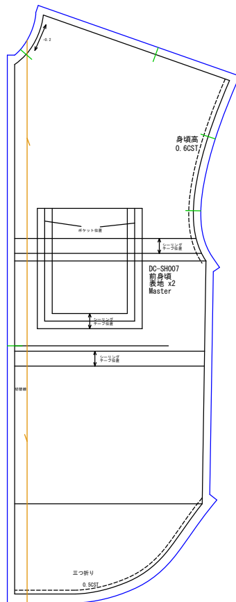
前身頃 表地x2
