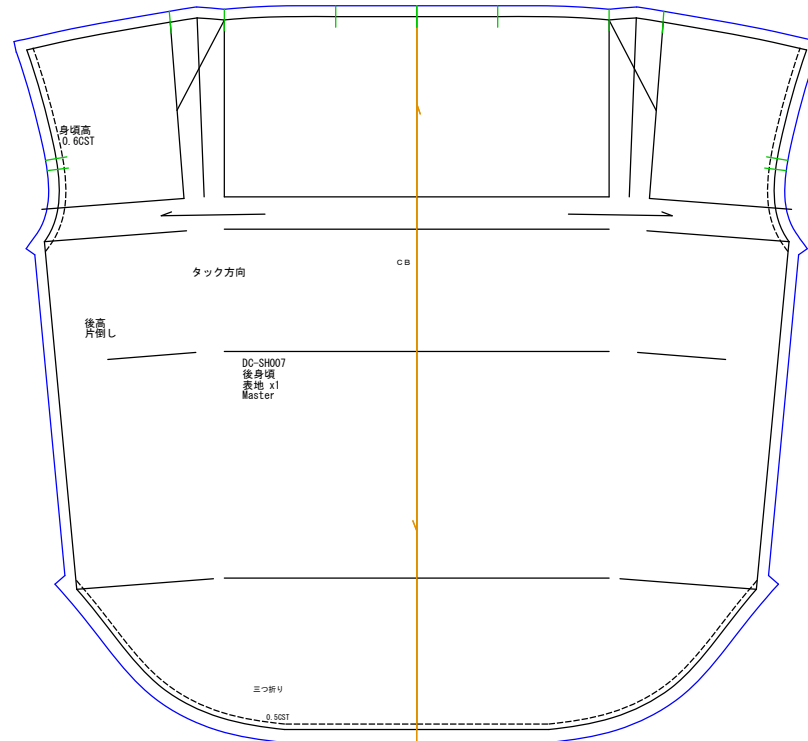
後身頃 表地x1
