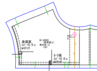
前身頃上 表生地x2
