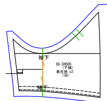
下袖 表生地x2
