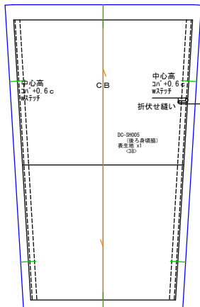
後ろ身頃脇 表生地x1
