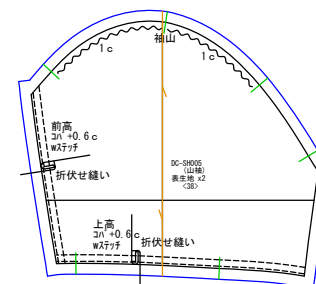
山袖 表生地x2
