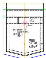
左前ポケット 表生地x1
