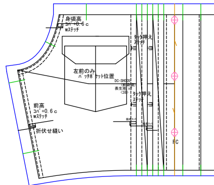
前身頃 表生地x2
