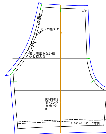
前パンツ 表地x2
