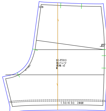
後パンツ 表地x2
