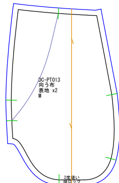
向う布 表地x2
