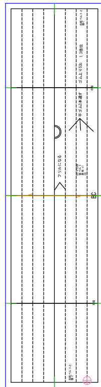
後ベルト 表地x1
