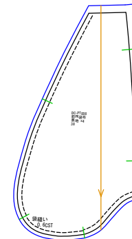
前PK袋布 表地x4
