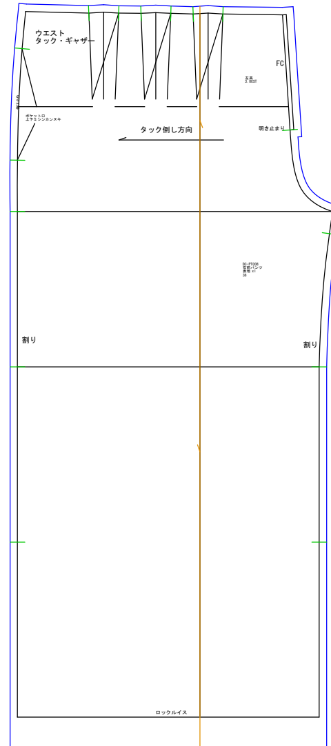
右前パンツ 表地x1
