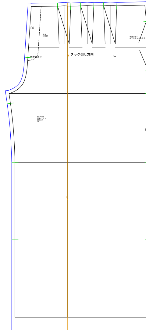
左前パンツ 表地x1
