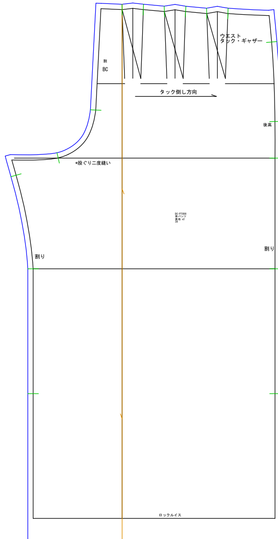
後パンツ 表地x2
