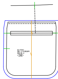
後* ヲット手前袋布 裏生地x2
