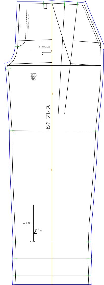
左前パンツ (1/7.4) 表生地x1 芯地x1
