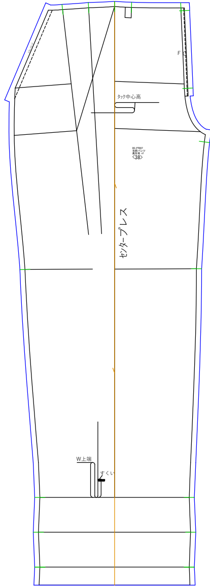
右前パンツ (1/7.4) 表生地x1
