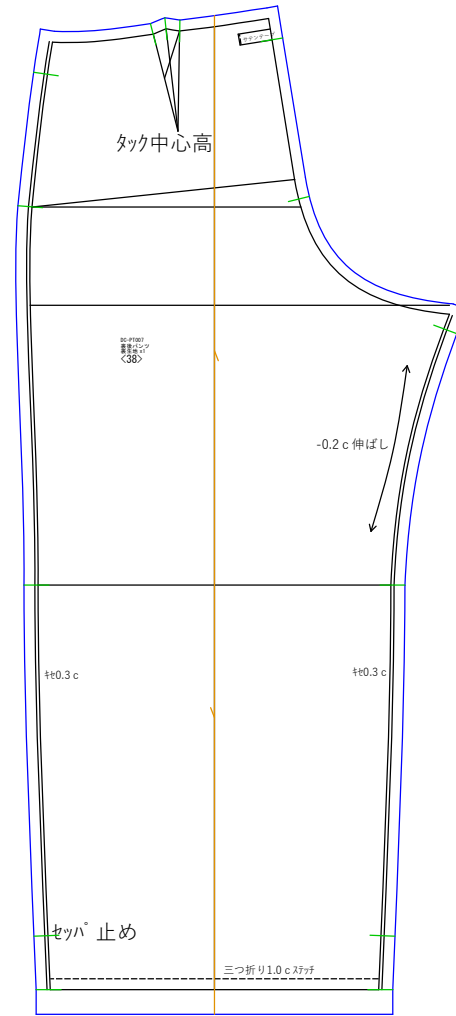
裏後パンツ 裏生地x1
