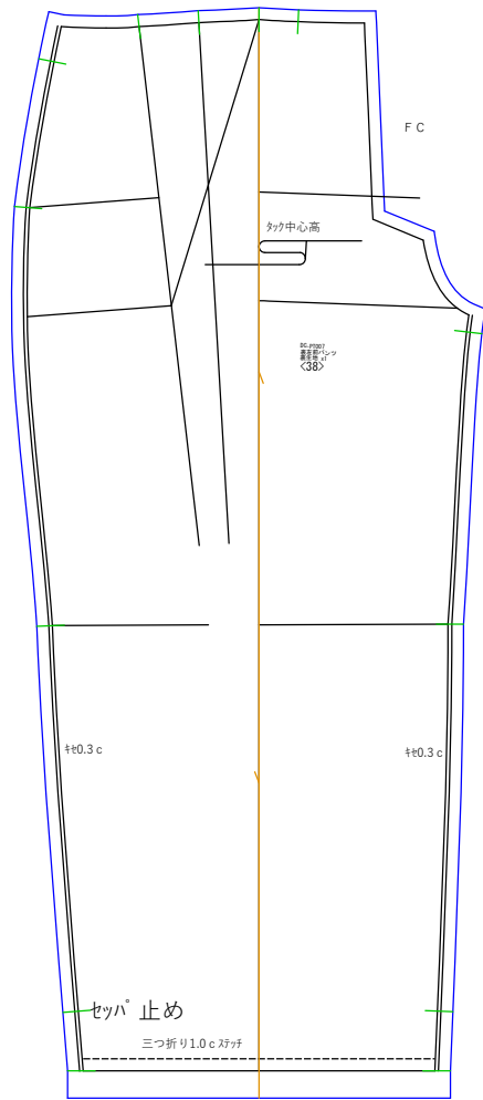
裏左前パンツ 裏生地x1
