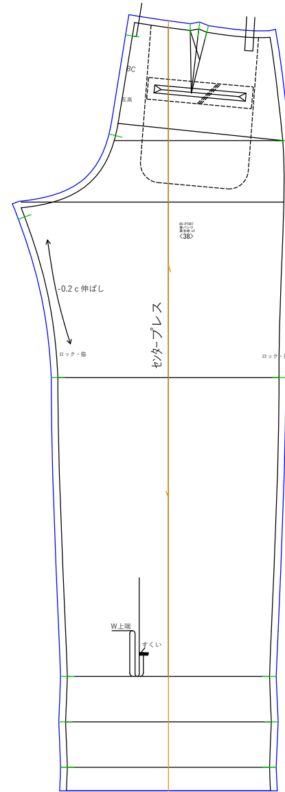
後* ヲット (1/7.7) 表生地x2
