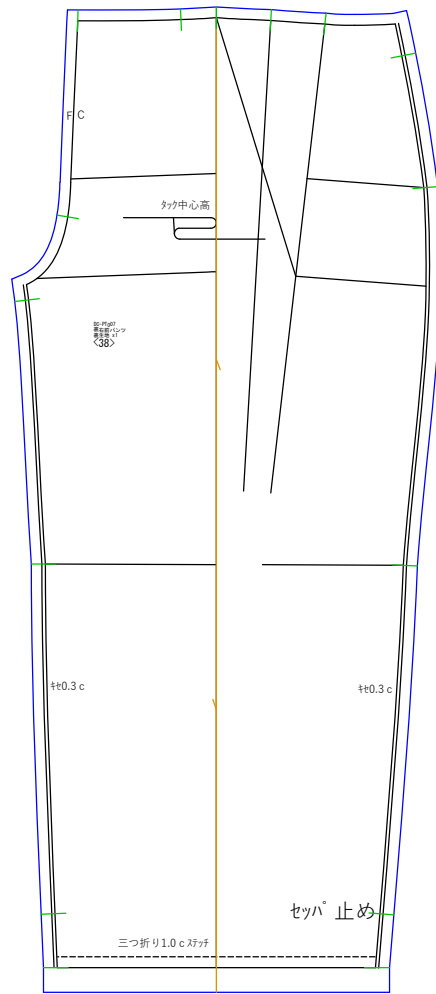
裏右前パンツ 裏生地x1
