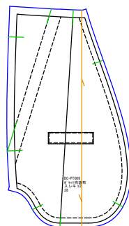
ポケット向袋布 スレキx2
