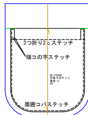
右後ろポケット 表地 x1
