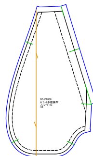
ポケット手前袋布 スレキx2
