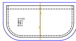
左フラップ 表地x2 芯地x2
