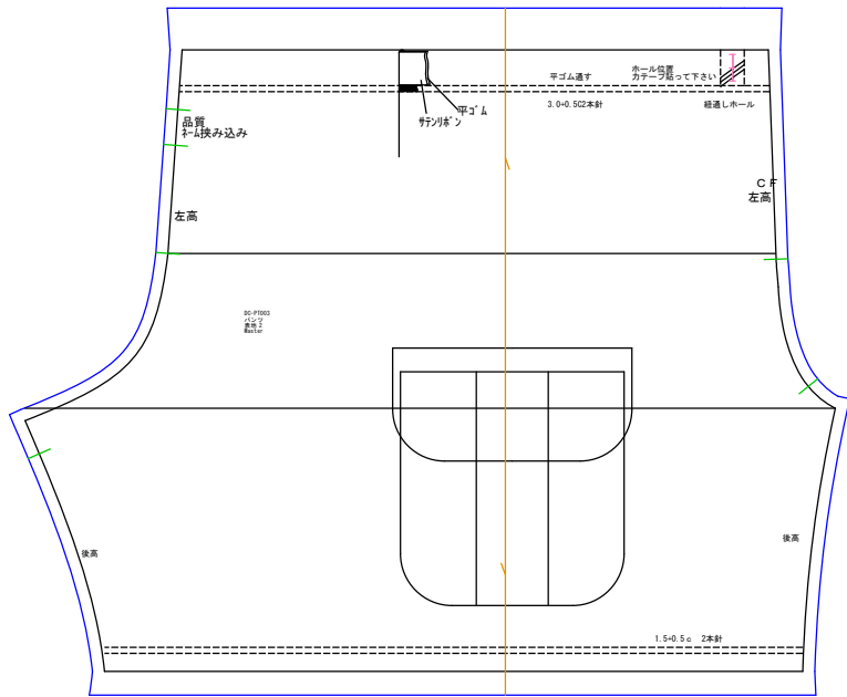
パンツ 表地x2
