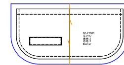
右フラップ 表地x2 芯地x2
