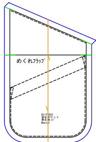
後右ポケット 表生地x1
