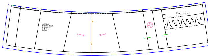
左前ウエスト見返し 表生地Bx1 芯地x1
