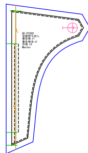
右前持ち出し 表生地x1 表生地B x1 芯地x2
