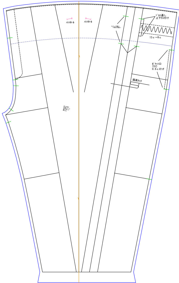
左前パンツ (1/7.0) 表生地x1
