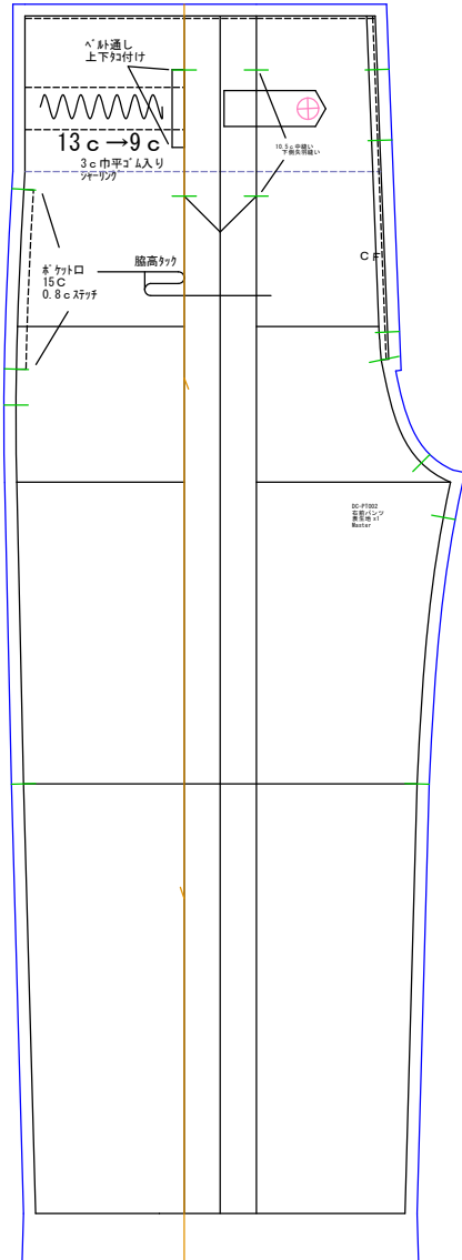
右前パンツ 表生地x1
