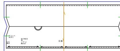
衿 リブx1
