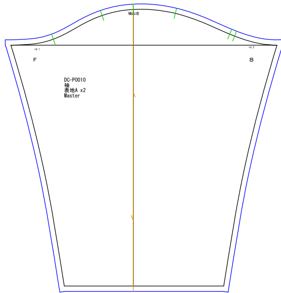
袖 表地Ax2
