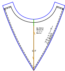
前汗止め リブx1
