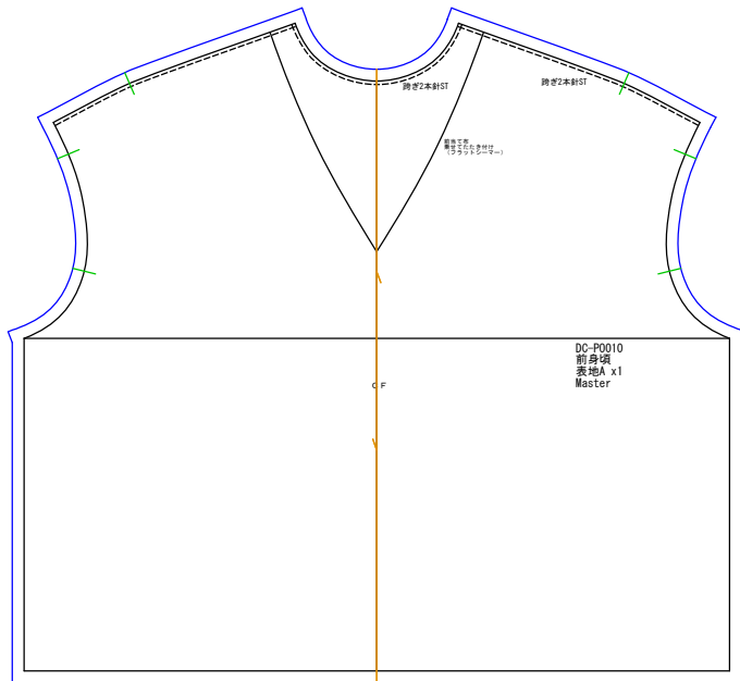
前身頃 表地Ax1
