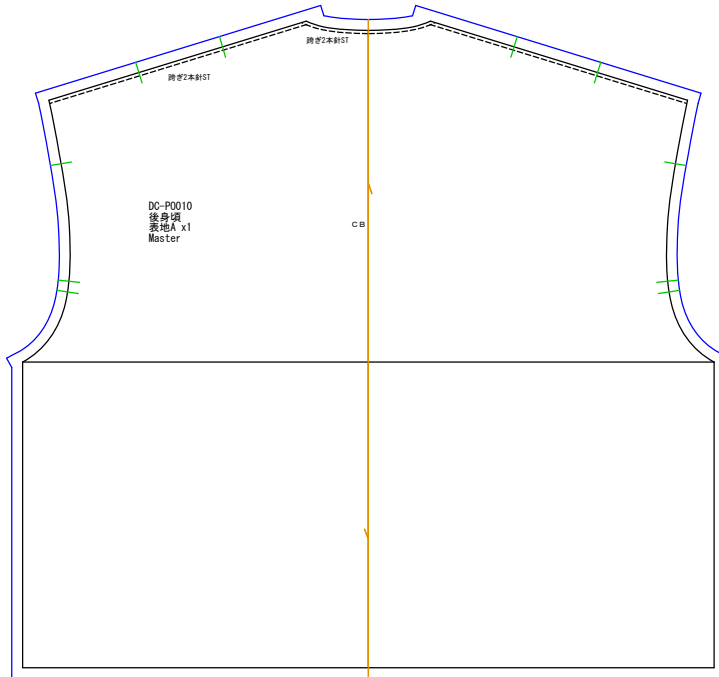
後身頃 表地Ax1
