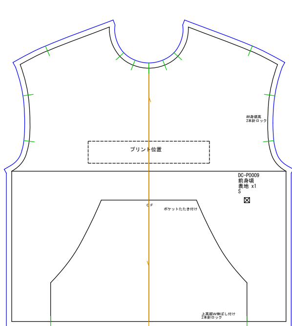
前身頃 表地x1
