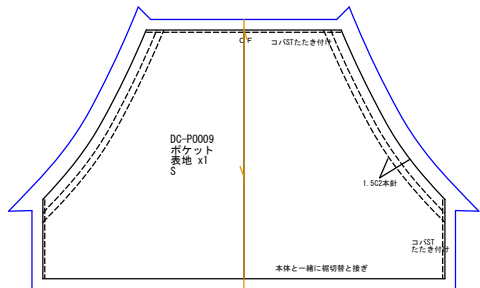
ポケット 表地x1
