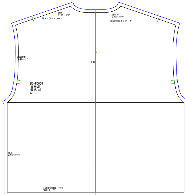
後身頃 表地x1
