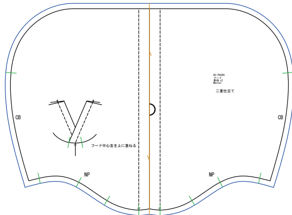
フード 表地x2
