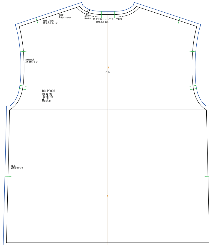
後身頃 表地x1
