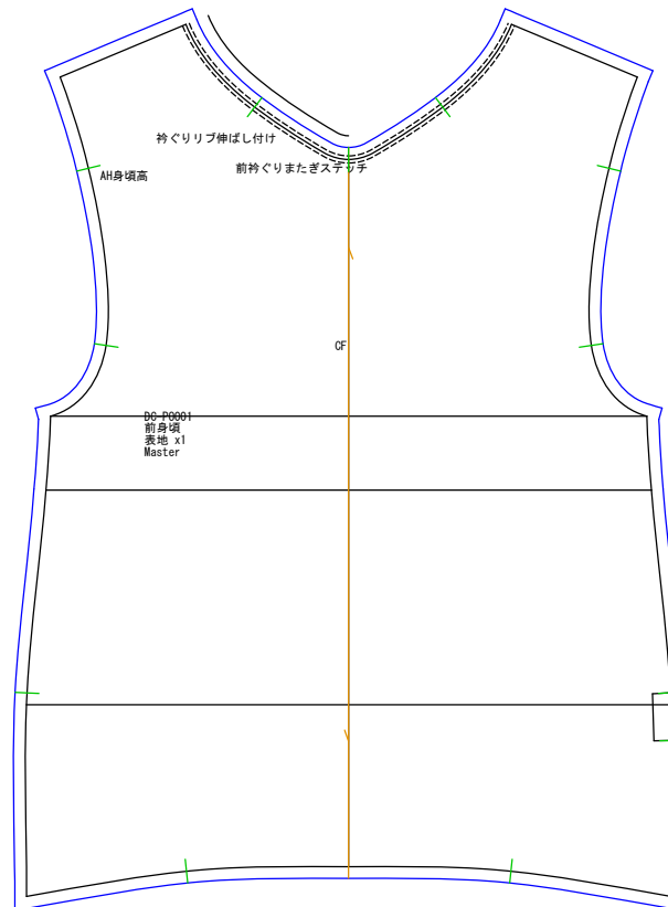
前身頃 表地x1
