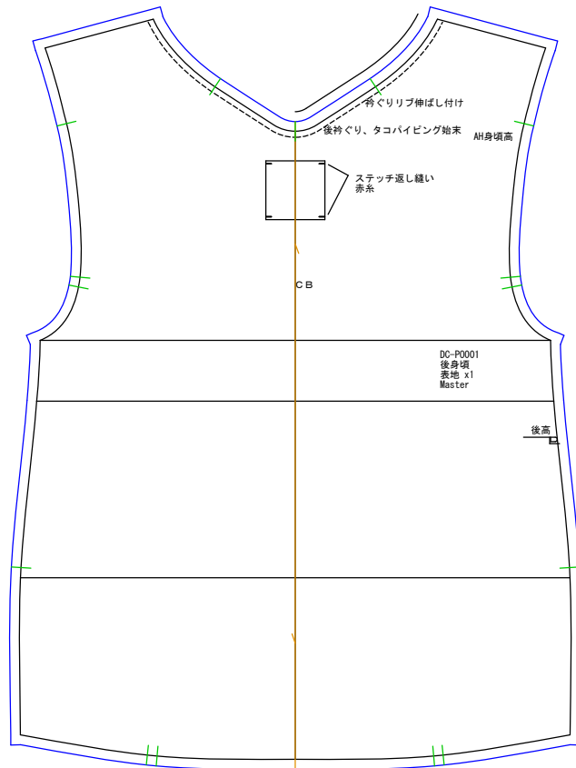
後身頃 表地x1
