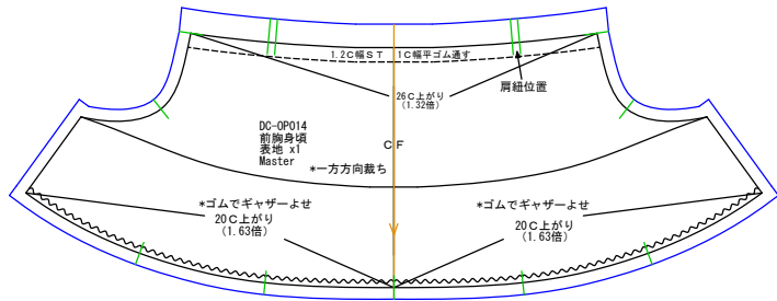
前胸身頃 表地x1
