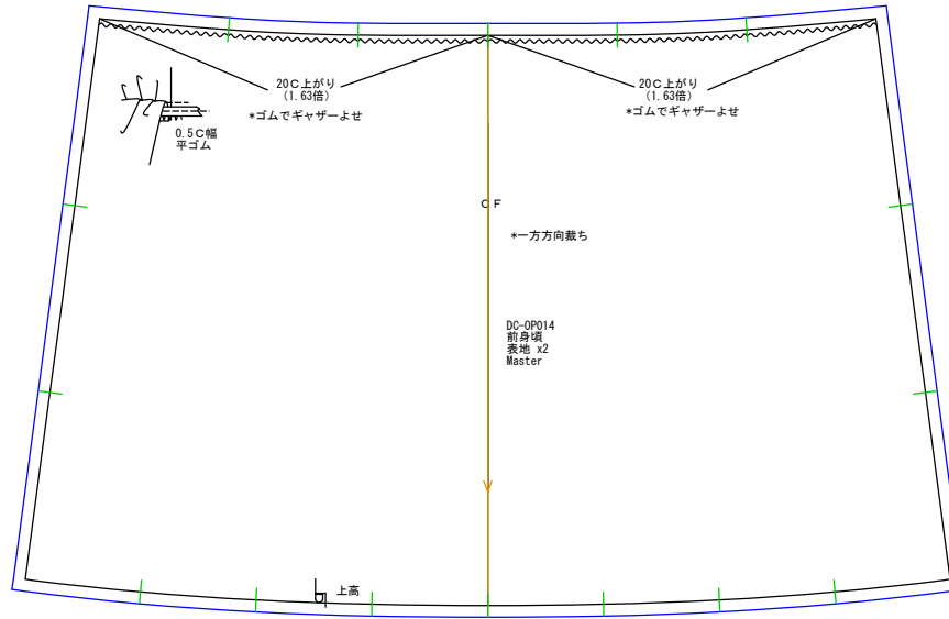
前身頃 表地x2
