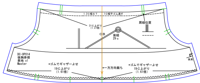
後胸身頃 表地x1
