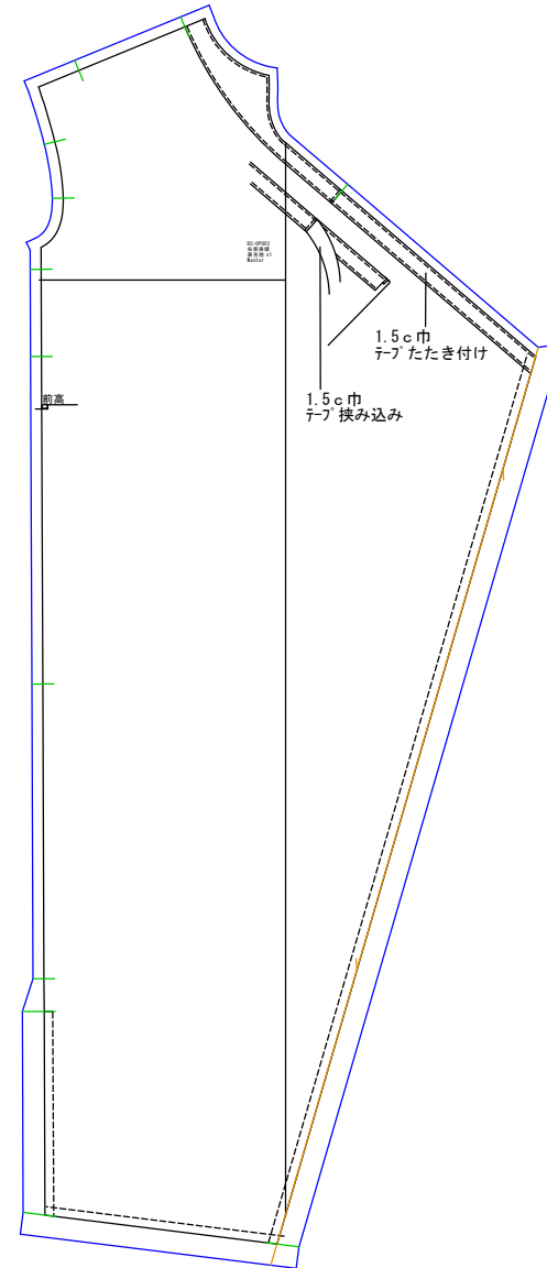
右前身頃 (1/7.6) 表生地x1
