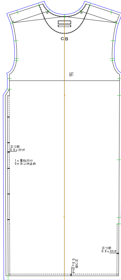
後身頃 (1/8.6) 表生地x1
