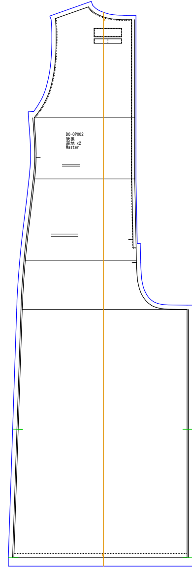
後身頃 (1/8.7) 裏地x2
