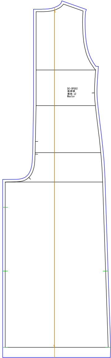
後身頃 (1/9.2) 表地x2
