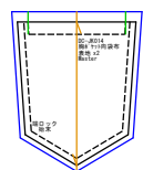
胸ホック向袋布 表地x2
