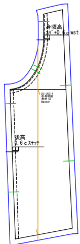
後身頃脇 表地x2
