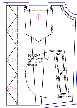
ホ ケットステッチゲージ ゲージx2
