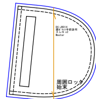
腰ホック手前袋布 スレキx2
