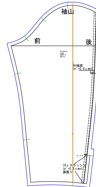
外袖 表地x2
