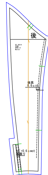
内袖 表地x2
