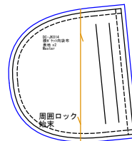
腰ホック向袋布 表地x2
