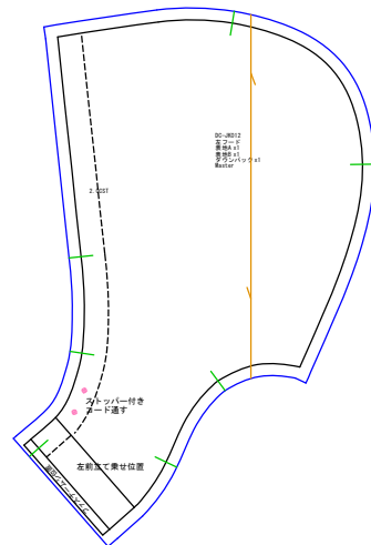
左フード 表地Ax1 表地Bx1 ダウンパックx1
