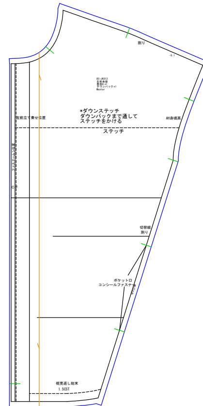
左前身頃 表地Ax1 ダウパックx1
