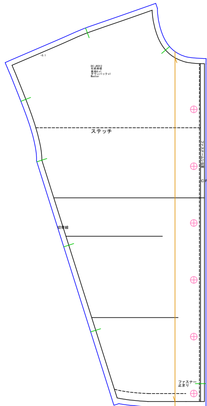
右前身頃 表地Ax1 ダウパックx1
