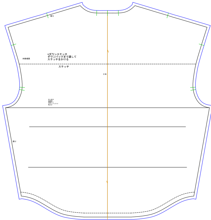
後身頃 表地Ax1 ダウンパックx1
