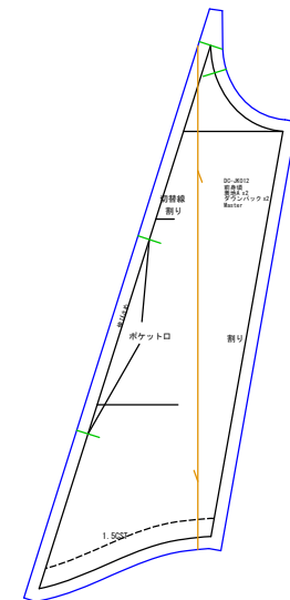
前身頃 表地Ax2 ダウパックx2
