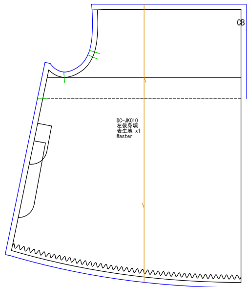
左後身頃 表生地x1
