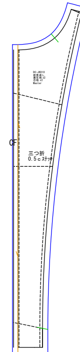
前見返し 表生地x2 芯地x2
