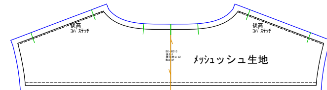
後ヨーク 表生地Cx2
