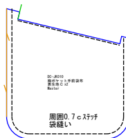
胸ポケット手前袋布 表生地Cx2
