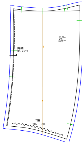
内袖 表生地x2
