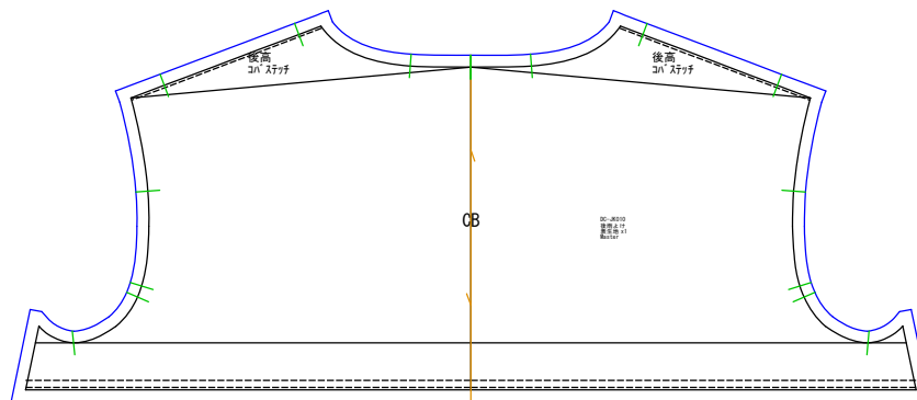
後雨よけ 表生地x1
