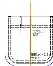
パッチポケット 表生地x2
