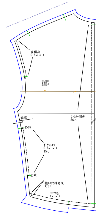
前身頃 表生地x2
