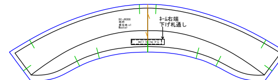
地衿 表生地 x1
