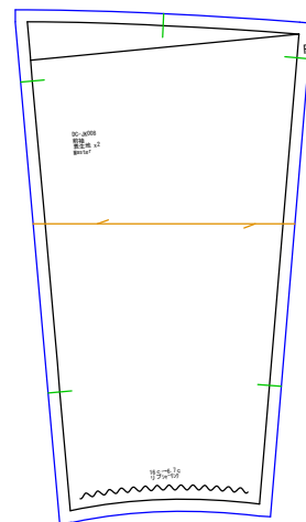
前袖 表生地 x2
