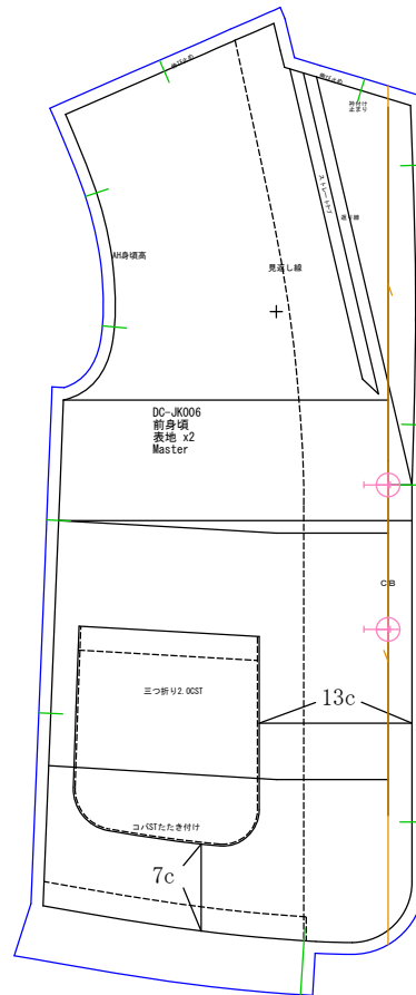
前身頃 表地x2
