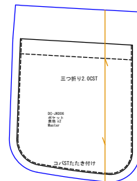
ポケット 表地x2
