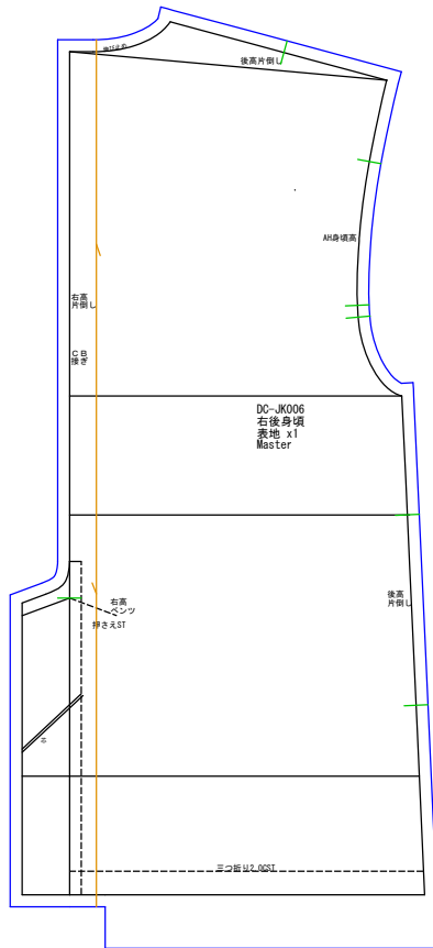
右後身頃 表地x1
