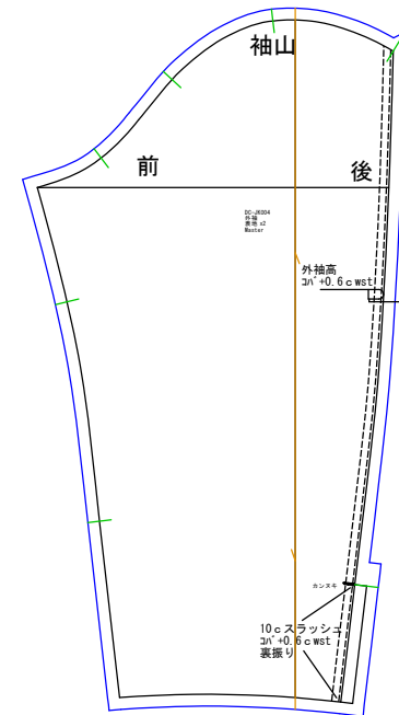
外袖 表地x2
