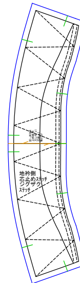
上衿地衿 スレキx1 芯地x1
