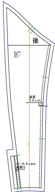
内袖 表地x2
