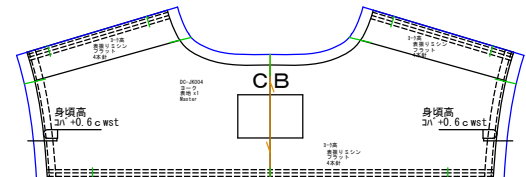
ヨーク 表地x1
