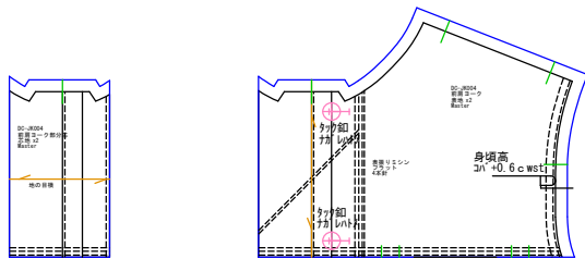
前肩ヨーク部分芯 芯地x2
