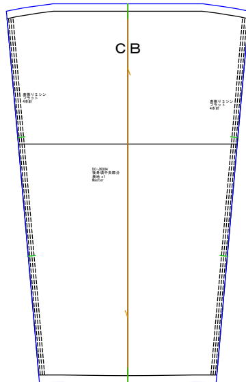
後身頃中央部分 表地x1
