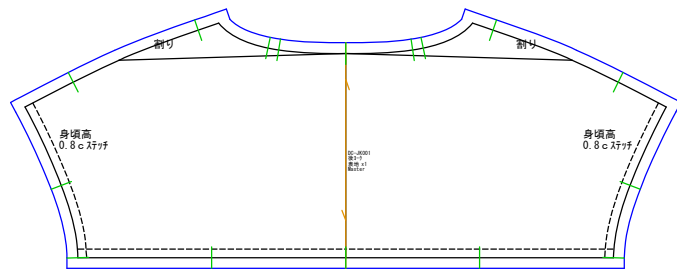
後ヨーク 表地x1
