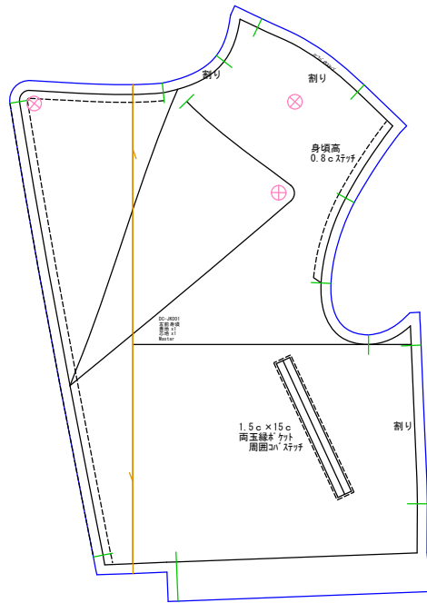
左前身頃 表地x1 芯地x1
