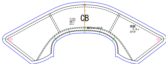
上衿表衿 表地x1 芯地x1
