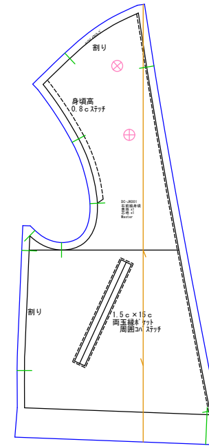
右前脇身頃 表地x1 芯地x1
