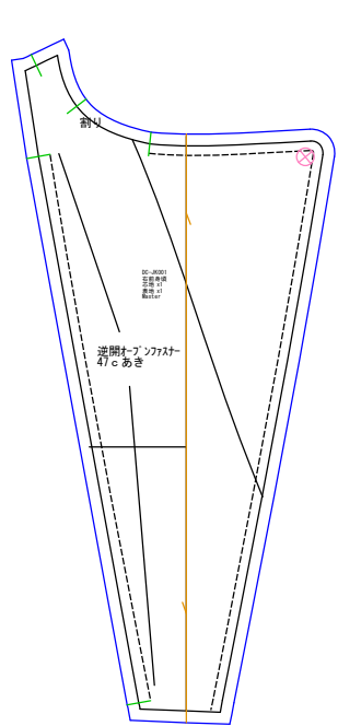
右前身頃 芯地x1 表地x1
