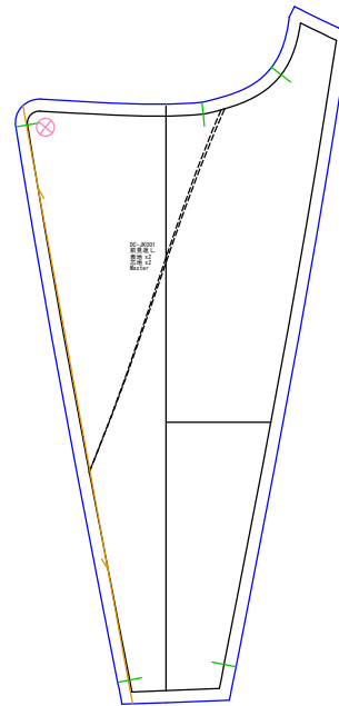
前見返し 表地x2 芯地x2
