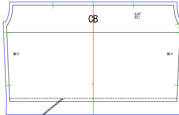
後身頃 表地x1
