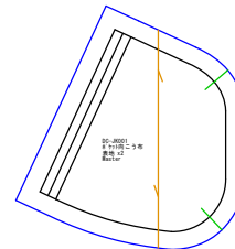
ポケット向こう布 表地x2
