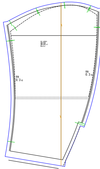
裏外袖 裏生地x2
