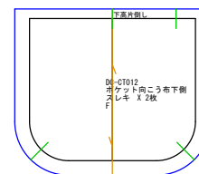
ポケット向こう布下側 スレキx2
