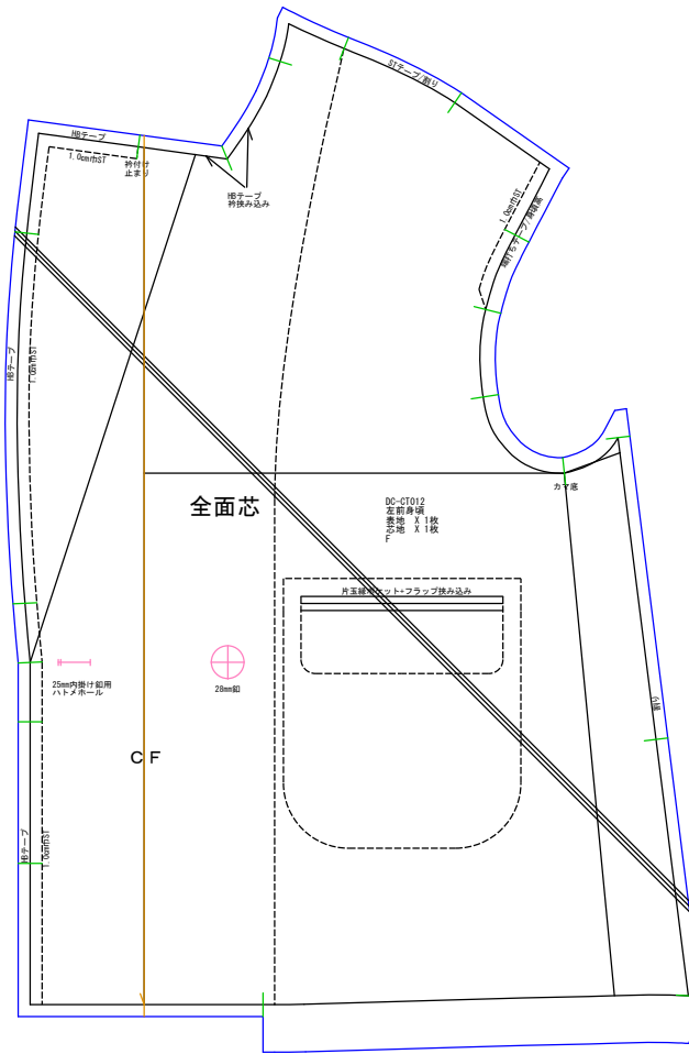
左前身頃 表地x1 芯地x1
