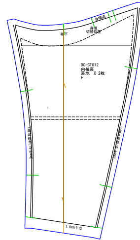
内袖裏 裏地x2
