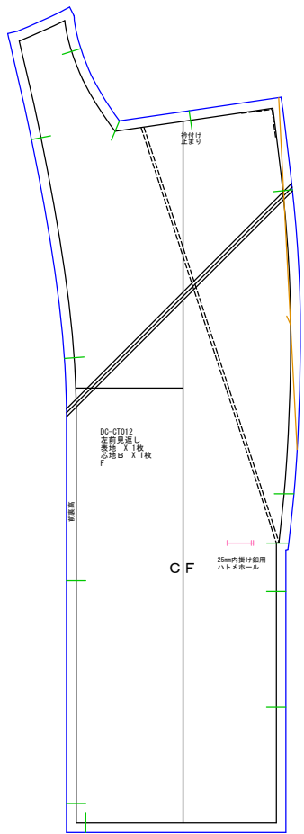
左前見返し 表地x1 芯地B x1
