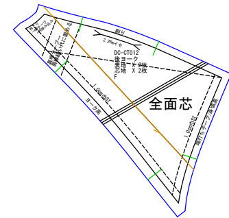
後ヨーク 表地x2 芯地x2
