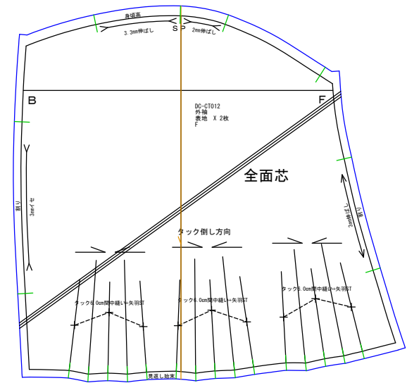
外袖 表地x2
