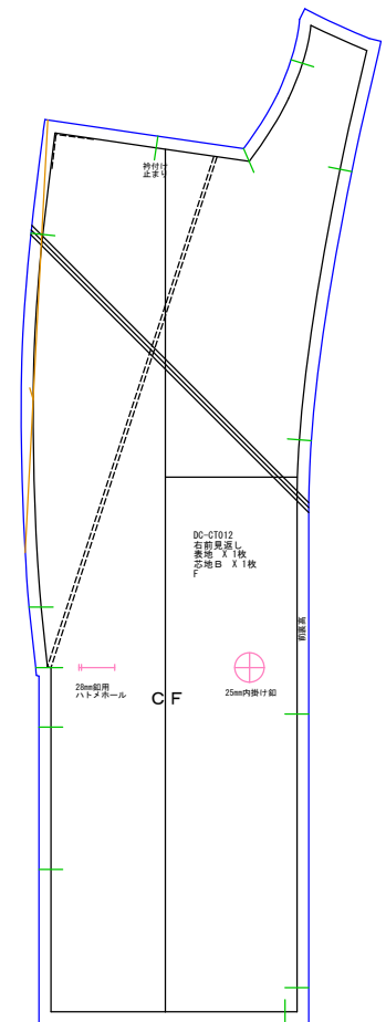
右前身見返し 表地x1 芯地Bx1
