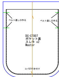
ポケット裏 スレキx2
