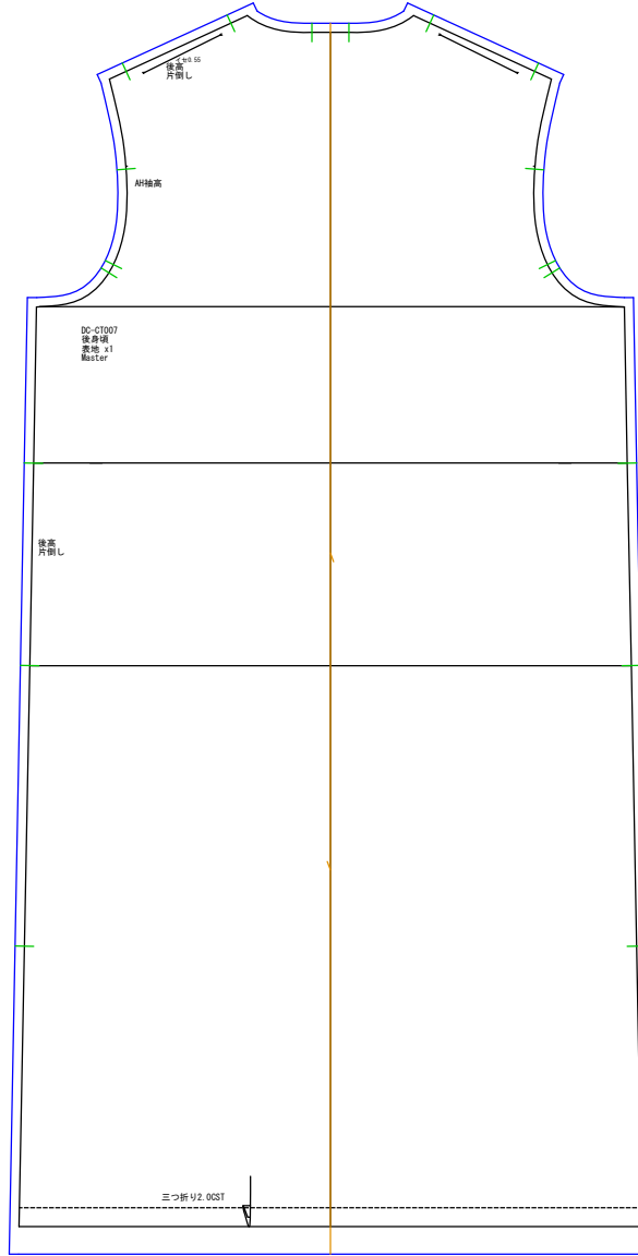
後身頃 (1/9.0) 表地x1
