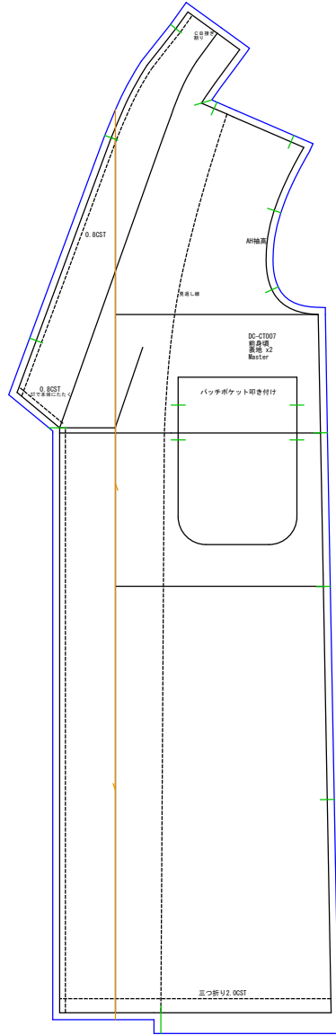
前身頃 (1/9.7) 表地x2
