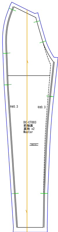
前袖裏 裏地x2
