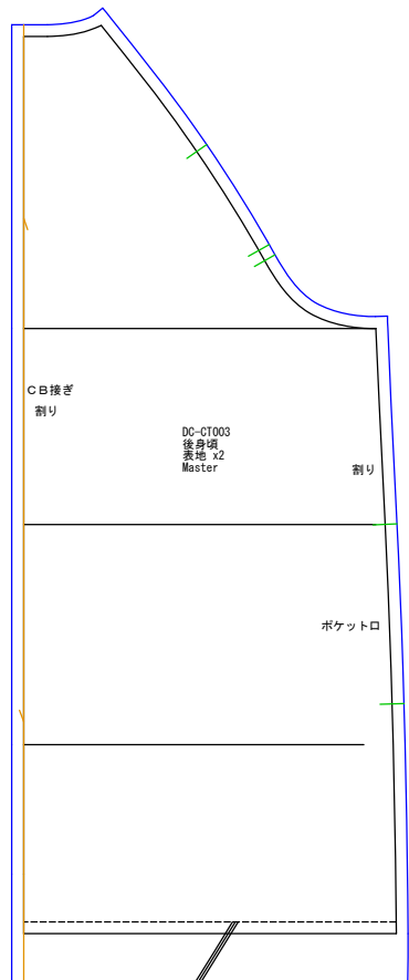
後身頃 表地x2
