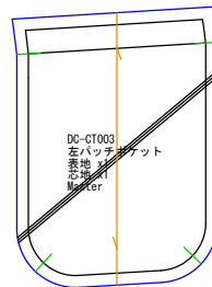
左パッチポケット 表地x1 芯地x1
