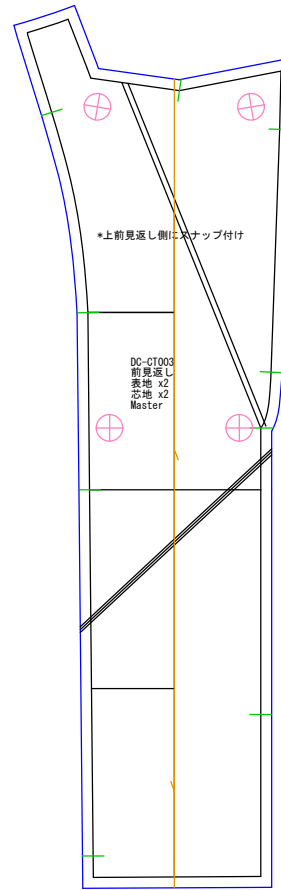
前見返し 表地x2 芯地x2
