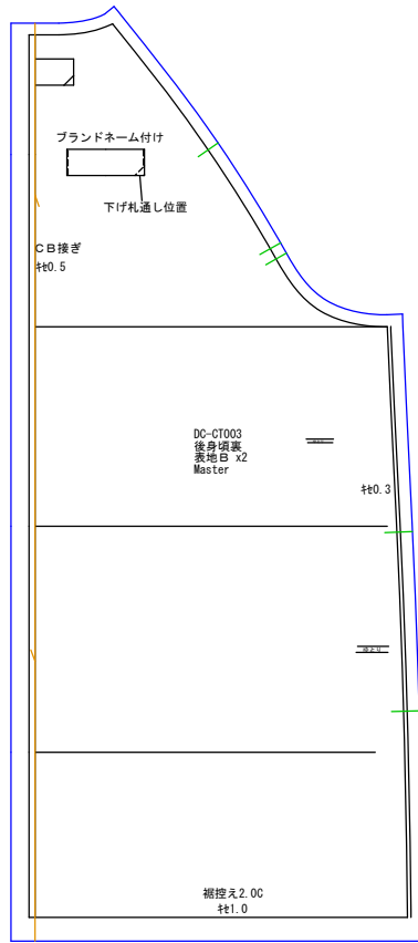
後身頃裏 表地 B x2
