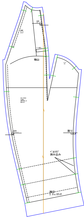
外袖 表生地x2
