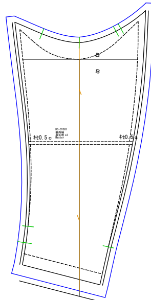
裏内袖 裏生地x2
