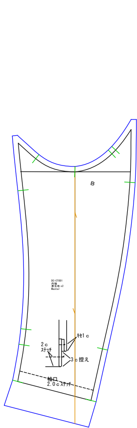
内袖 表生地x2
