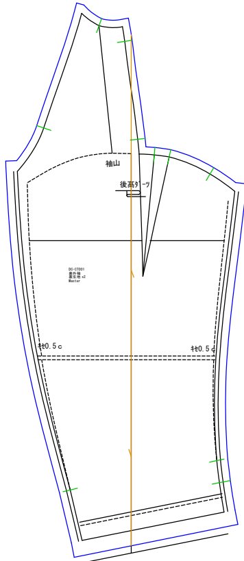
裏外袖 裏生地x2
