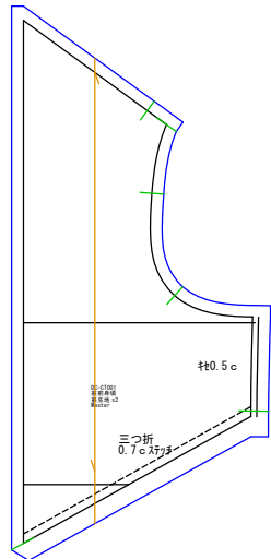
裏前身頃 裏生地x2
