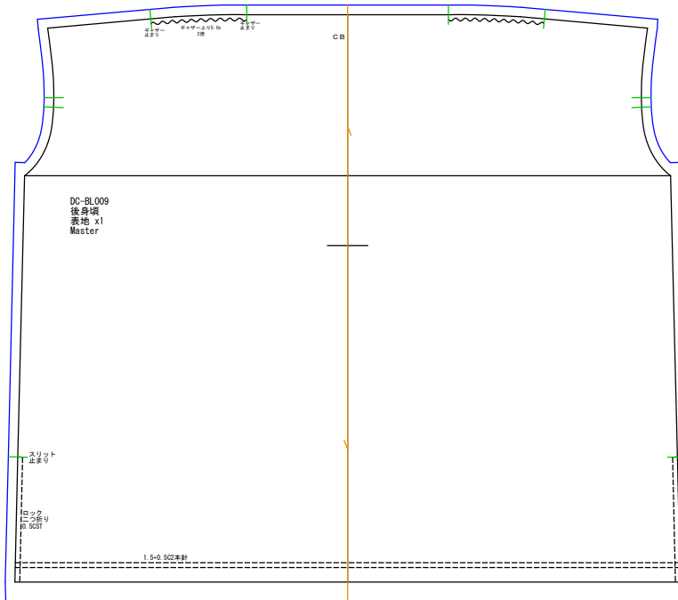
後身頃 表地x1
