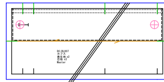
カフス 表生地x2 芯地x2
