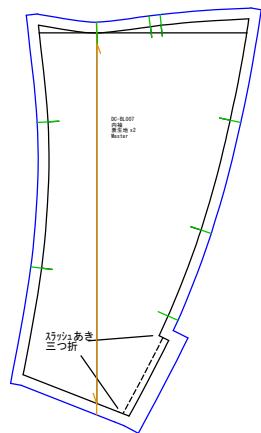
内袖 表生地x2
