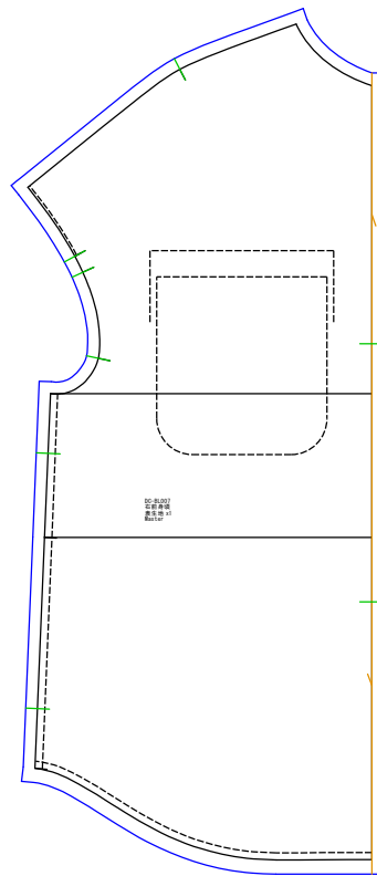
右前身頃 表生地x1
