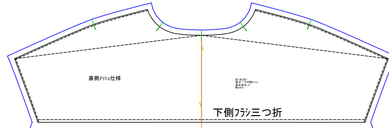
後ヨーク内側メッシュ 表生地B x1
