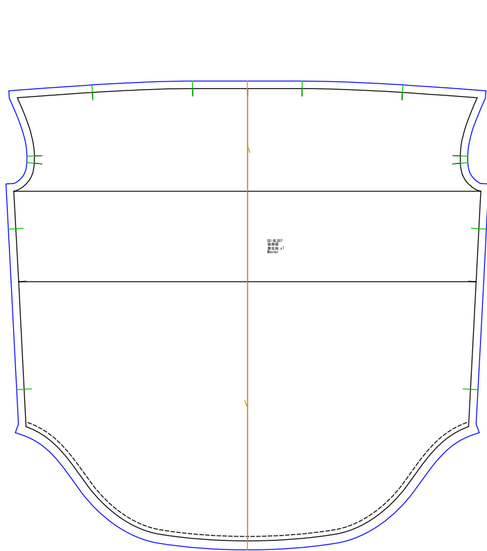
後身頃 表生地x1
