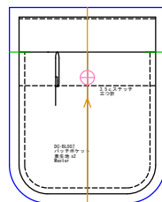
パッチポケット 表生地x2
