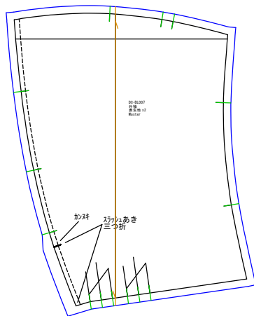
外袖 表生地x2
