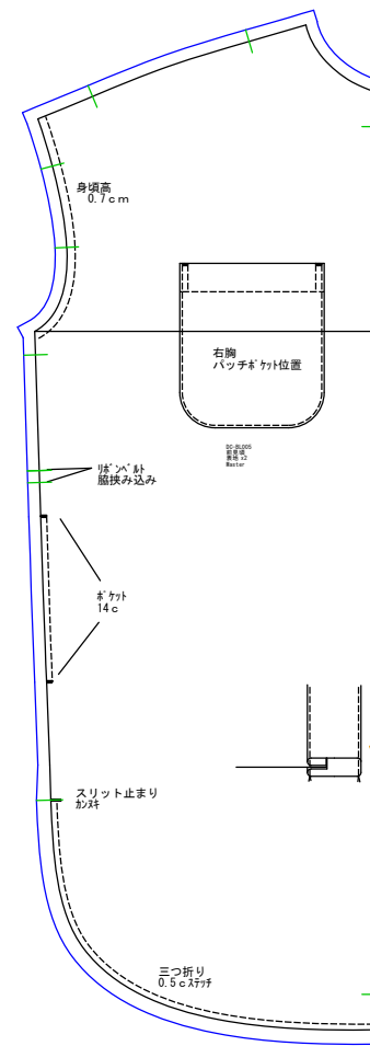
前見頃 表地x2
