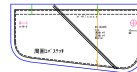
カス 表地x4 芯地x4
