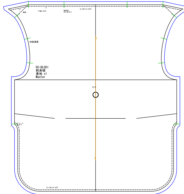
前身頃 表地x1
