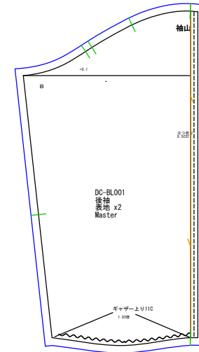
後袖 表地x2
