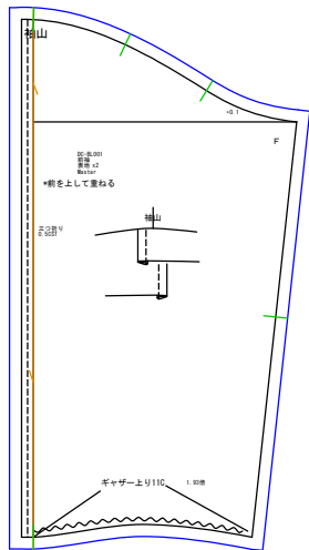
前袖 表地x2
